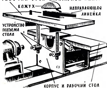
РАБОЧИЙ СТОЛ ЦИРКУЛЬНОЙ ПИЛЫ
