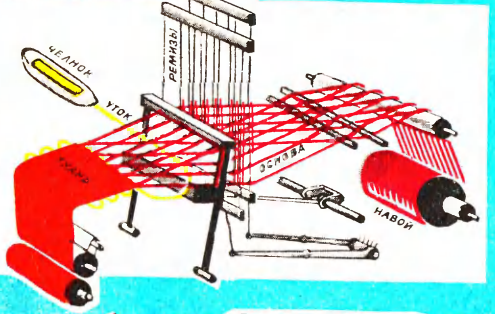
ТКАЦКИЙ СТАНОК
